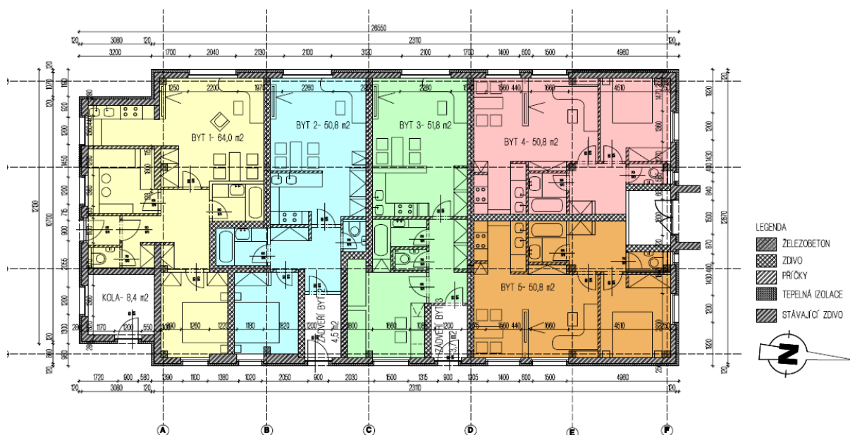
PŮDORYS 1.NP M 1: 100
